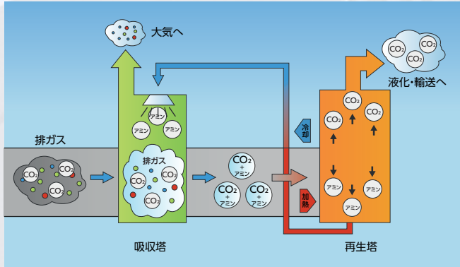
火力発電所からの排ガスがアミン溶液と触れることで、アミンがCO 2 を吸収。これを加熱することで、アミンとCO 2 が分離し、高濃度のCO 2 を回収することができます。
